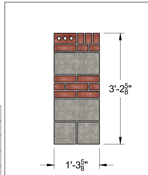
3. LEFT END
